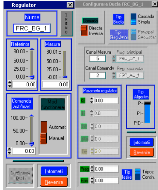
Fig. 2. FRC-1 – Control module
